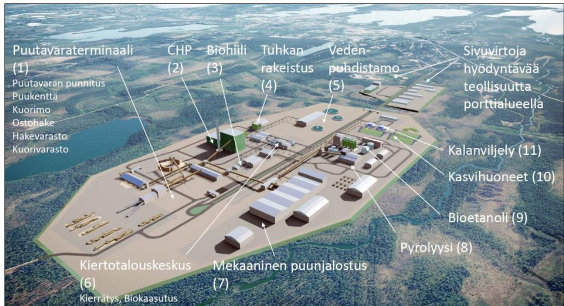
Kuva 3. Masterplanin layout ja toiminnot.
