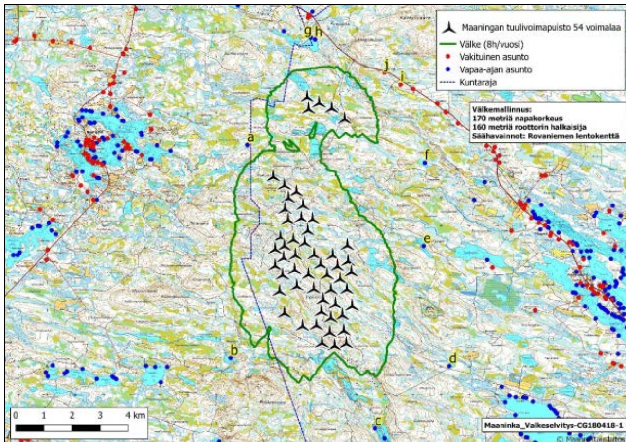
Kuva 9.20. Varjovälkkeen muodostuminen. Väkeraja (8 tuntia/vuosi) on merkitty vihreällä viivalla. Kuvaan on merkitty havainnointipisteet (a-j).
