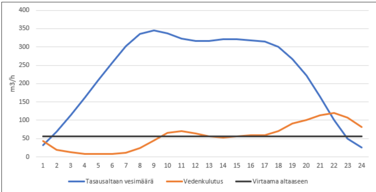
Kuva 4.1. Tasausaltaan vesimäärä ja vedenkulutukset arvioidun suurimman vuorokausikulutuksen aikana.
