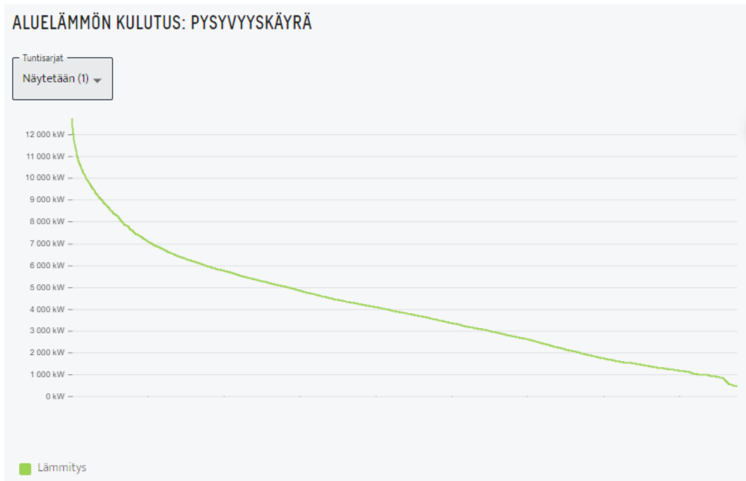
Kuva 6.2 Uudiskohteiden lämmitysenergiatarpeen pysyvyyskäyrä. Huipputehontarve on hyvin hetkellinen.
